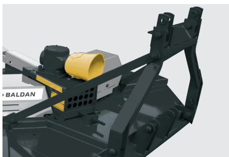
Cabeçalho de engate com regulagem para trabalhar na posição lateral e super lateral. Hitch with lateral and extend mounted adjustment. Barra de enganche que permite regular el equipo para trabajos en las posiciones lateral y super lateral.
